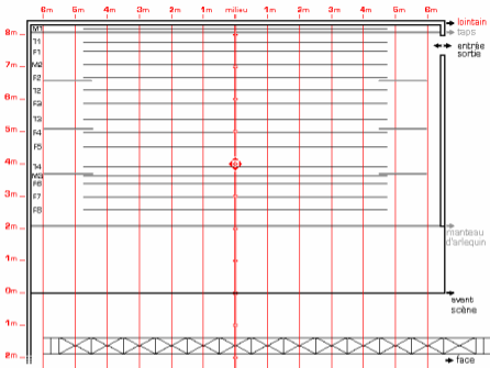
PLAN DE FEU échelle: 1/75ème
